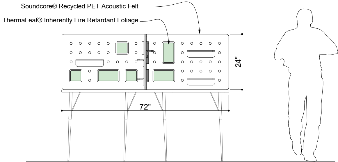
① ELEVATION 1
