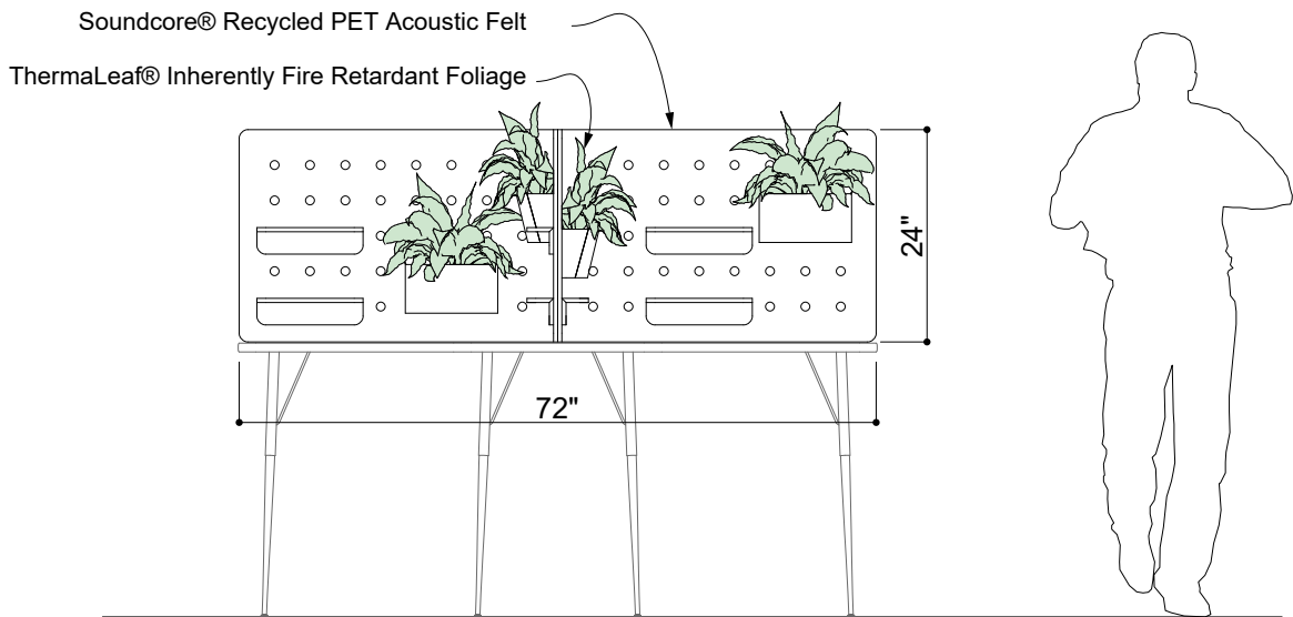
② ELEVATION 2
